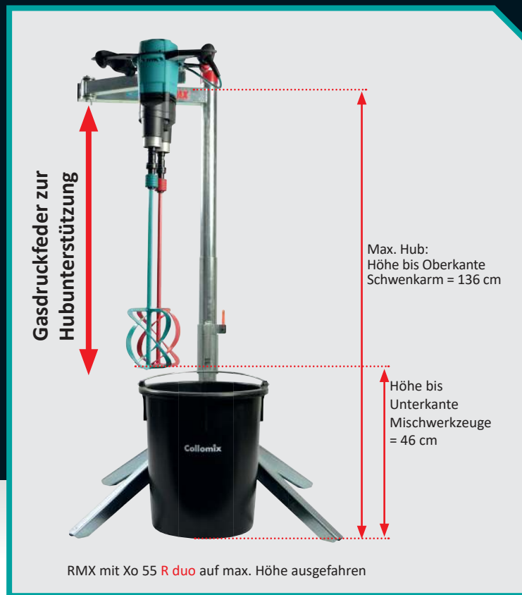
RMX mit Xo 55 R duo auf max. Höhe ausgefahren Lieferumfang Rührständer RMX ohne Maschine und Eimer
